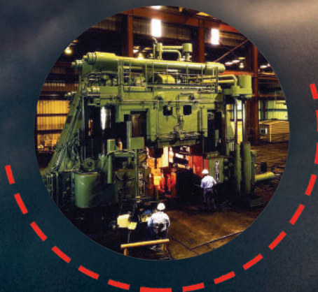
11,000 Ton Multi-ram Press
